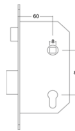
Cerradura YDI (desbloqueo interior)
