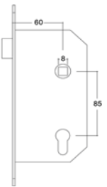
Cerradura anti pánico con trinco
