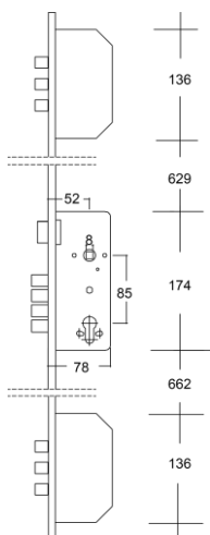
Serrure de sécurité avec 3 points
