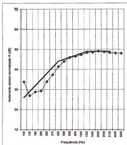
R_{w} (C; C_{125}; C_{500}; C_{1000}) = 45 (-2; -6; -1; -6) dB (Resultados obtenidos de acuerdo con la norma NP EN ISO 717-1:2009)
