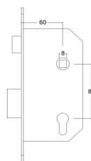
Cerradura YSE (salidas emergencia)
