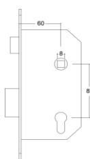
Cerradura YDI (desbloqueo interior)
