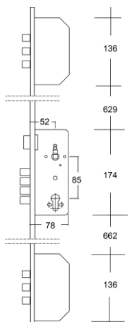
Serrure de sécurité de 3 points
