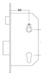
Fechadura YSE (saídas emergência)
