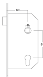
Fechadura trinco
