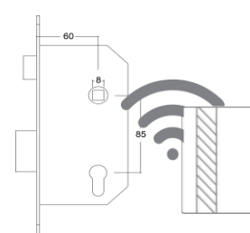
Fechadura YSE (saídas emergência)
