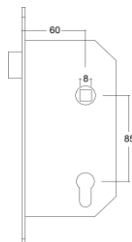
Fechadura trinco
