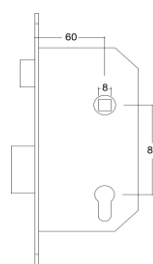
Serrure yale YDI (débloqué intérieur)
