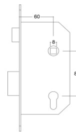
Serrure yale YSE (sorties de secours)
