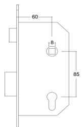
Fechadura YDI (desbloqueio interior)
