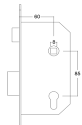
Fechadura YSE (saídas emergência)
