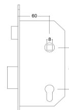
Serrure yale YSE-sorties de secours YDI- déblocage intérieur
